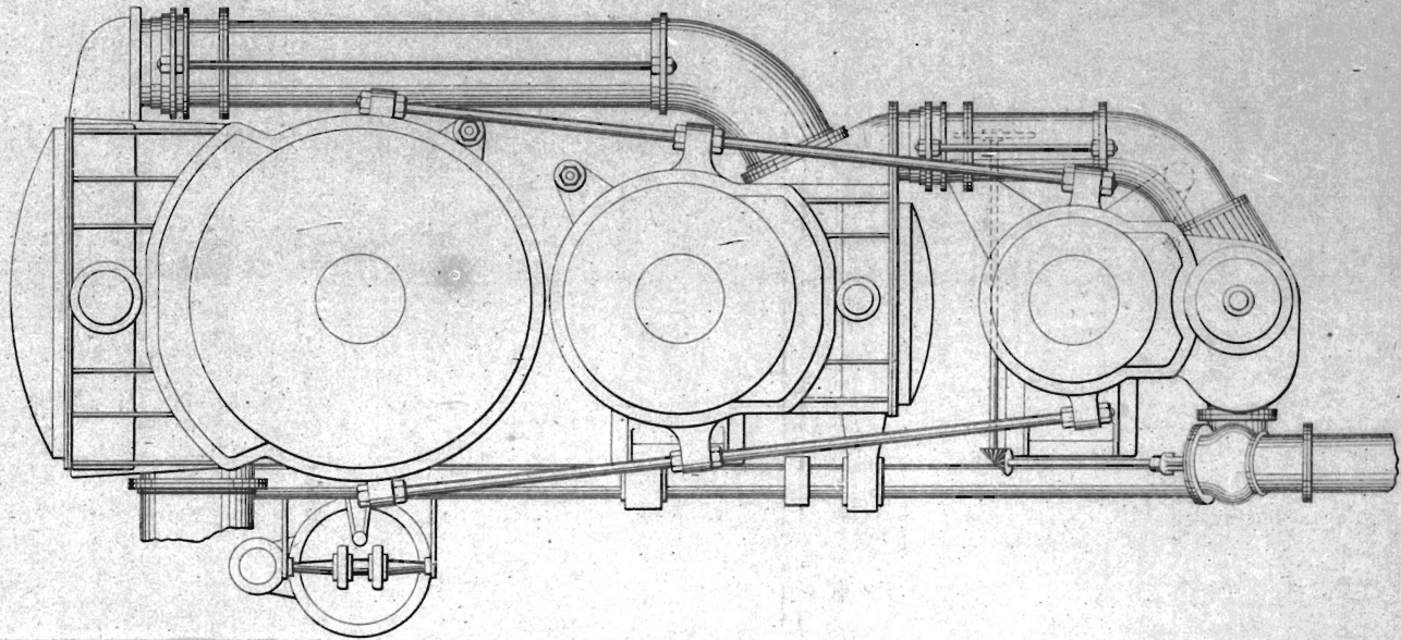
Navy Engines. Fig. 24. Plan.
