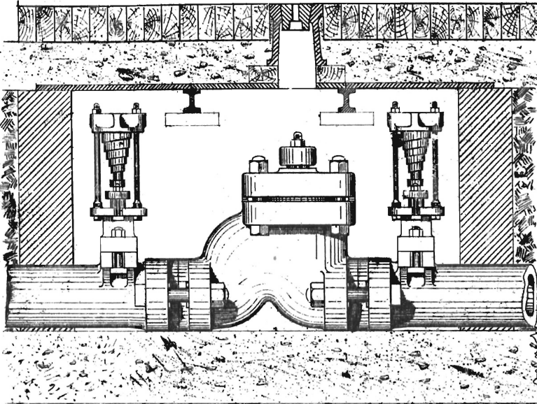
SECTION LONGITUDINAL
